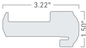
ASTRAGAL
